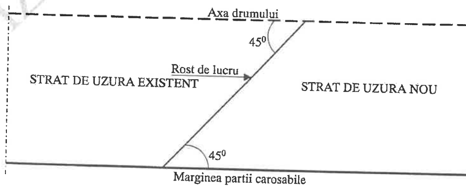
Fig. 1 Racordarea in plan a stratului nou cu stratul existent
